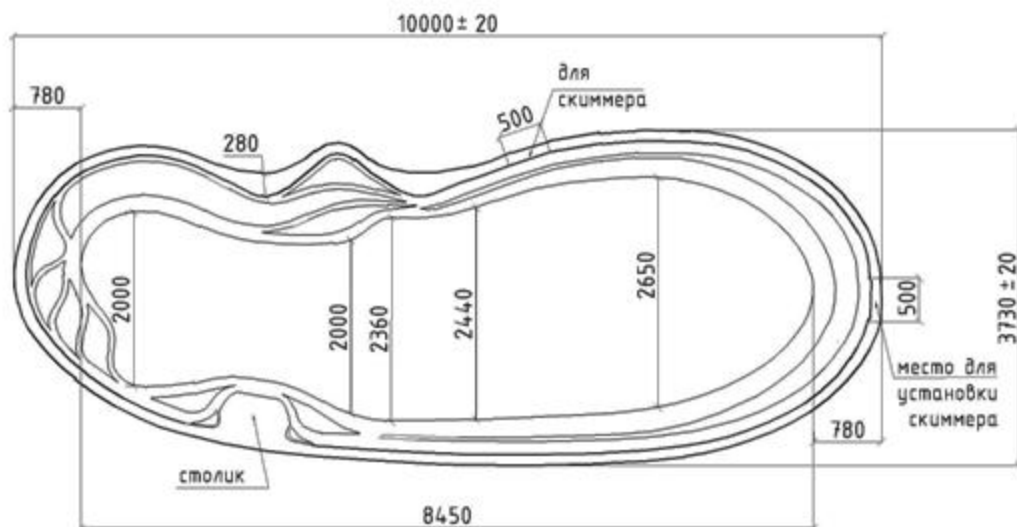
← Вид-А
