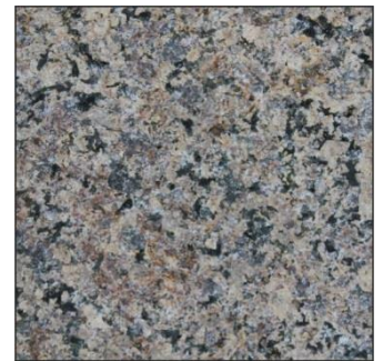
ДЕСЕРТ БРАУН
