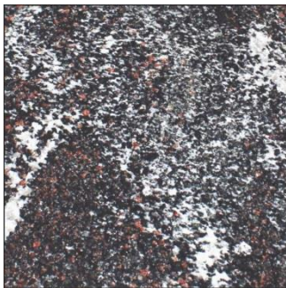
АМФИБОЛИТ
